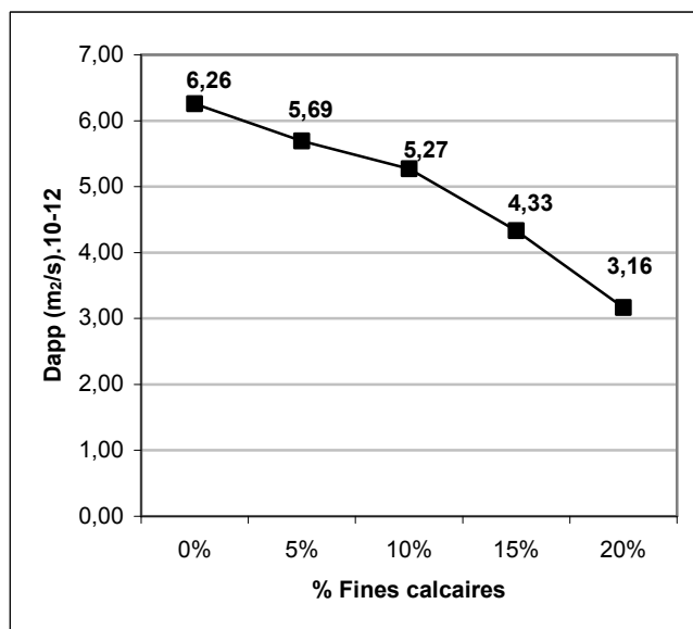
Fig. 6. Essai de migration des ions de chlorures
