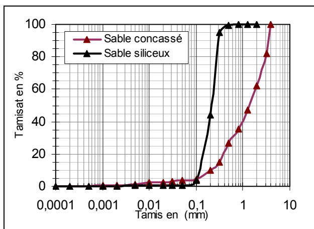
Fig. 1. Courbe granulométriques des SC et SS
